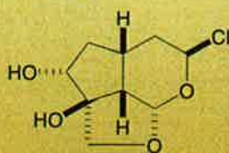
Kankanol
